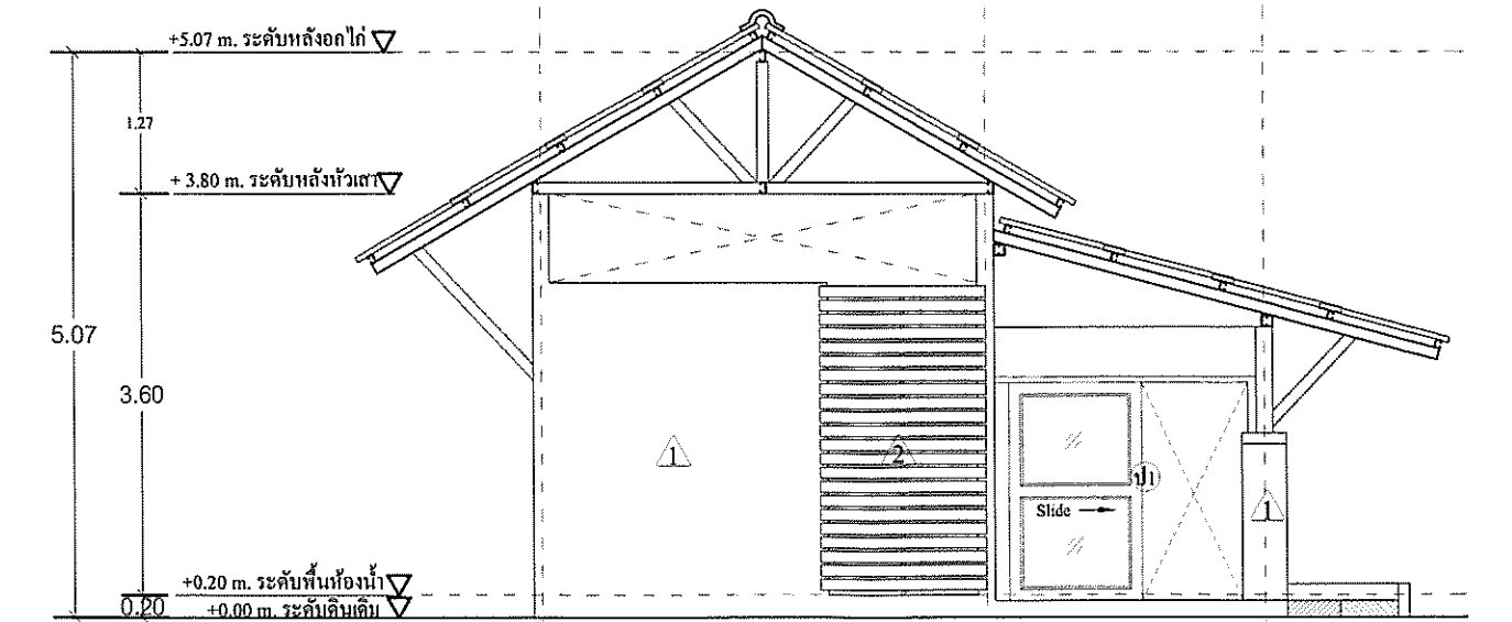
รูปด้าน D มาตรฐาน 1:75 (ห้องน้ำ)
