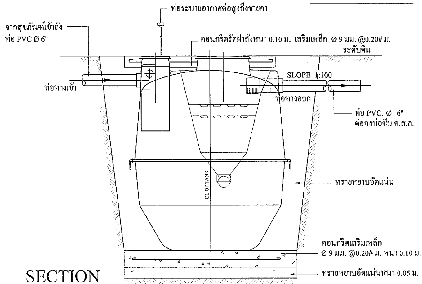
แบบขยายถังบำบัดน้ำเสีย
