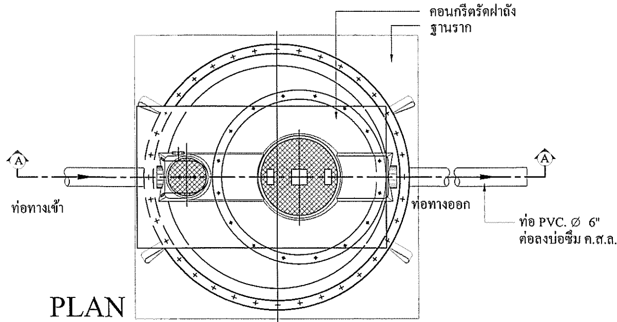
แบบขยายถังบำบัดน้ำเสีย
